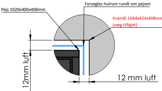
DK - View D 1:2
